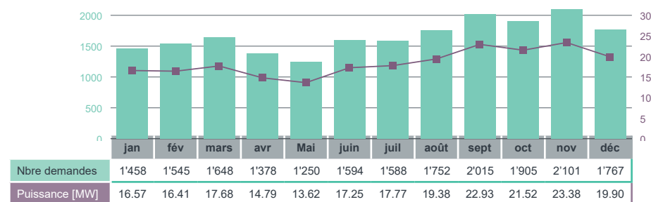
Diagramme 4: Réception des demandes PRU 2021 - catégorie de puissance < 30 kWc
